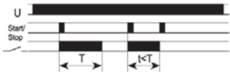
FZ38: anzugsverzögert mit Start/Stop-Taste
