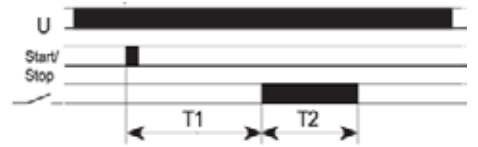
FZ41: Impulsgeber mit Start/Stop-Taste
